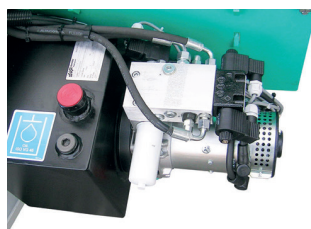
Centralina idraulica
